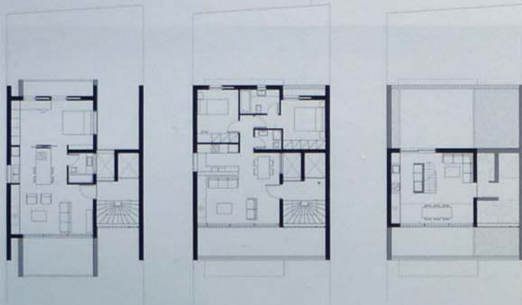
Κατοψη πρώτη και δεύτερου ορόφου First and second floor plan
